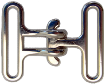
イカリ引掛カン 30 mm (Z)ニッケル 箱 /200 ケ◎ イカリ / 全長 26× 幅 37× 内径 31 mm 受け / 30× 37× 31 mm
