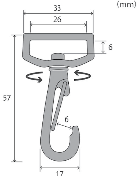
太網ナスカン OK-24(Z)ニッケル 亜鉛合金(バネ:鉄製) 箱/400 ケ
