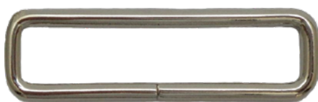
コカン 50×10×3.5(A)ニッケル 幅(内)51×高(内)10 mm 箱/400 ケ
