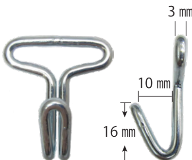
引掛カン 3×25(A)ニ加 ロー付 全長 34× 幅 31× 内径 25 mm 箱 /400 ケ◎
