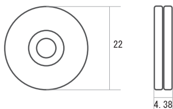
寸法図（組立時）
